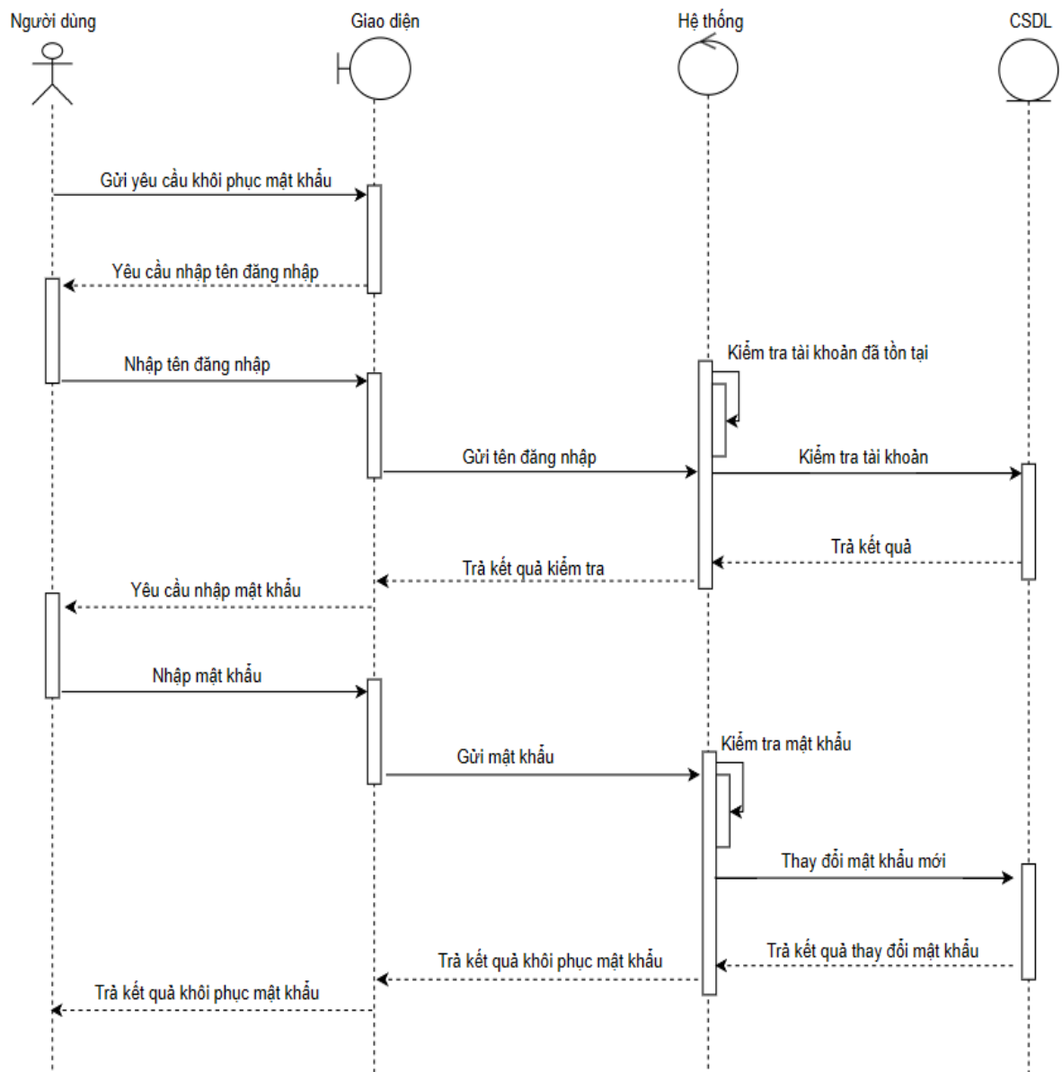
Hình 6: Sơ đồ trình tự khôi phục mật khẩu
