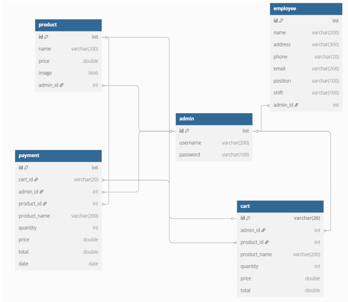
Hình 22: Mô hình ERD (Entity-Relationship Diagram)
