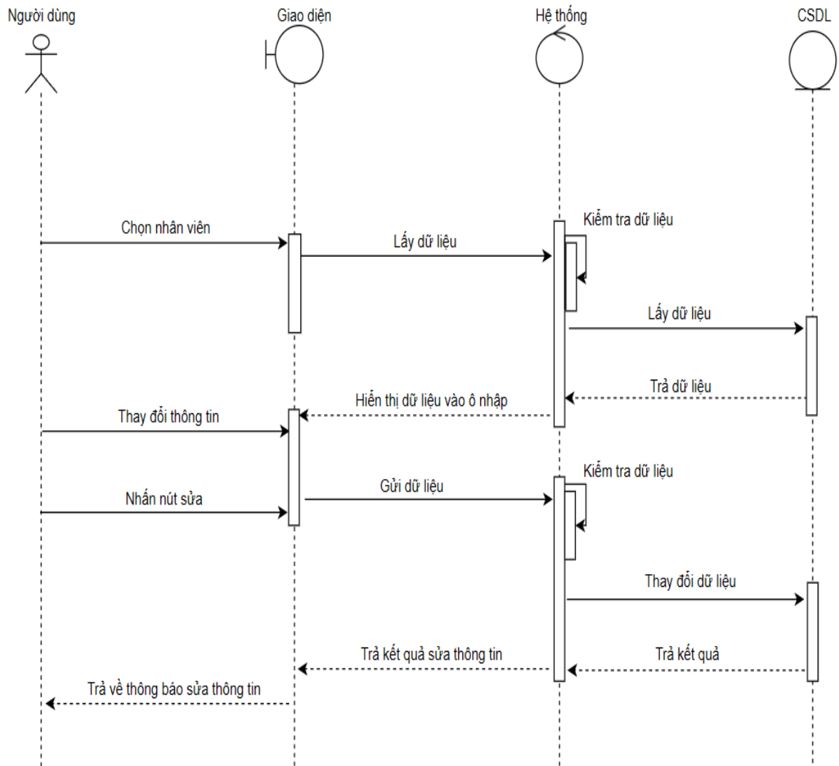
Hình 18: Sơ đồ trình tự sửa thông tin nhân viên
