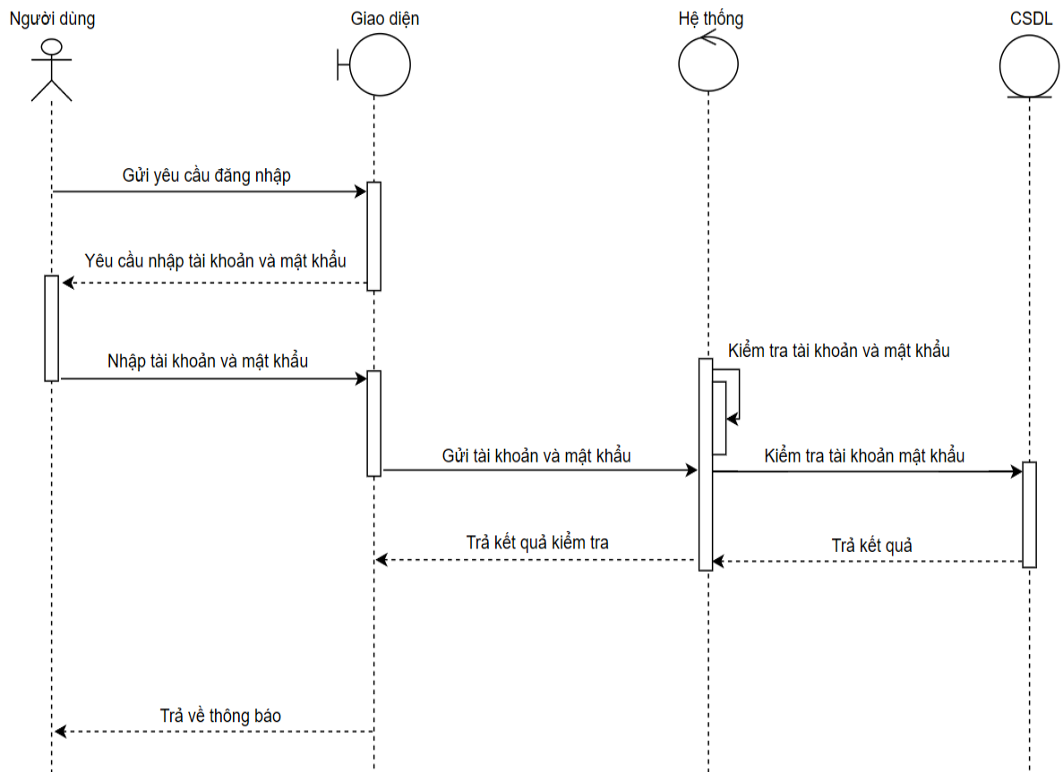
Hình 4: Sơ đồ trình tự đăng nhập
