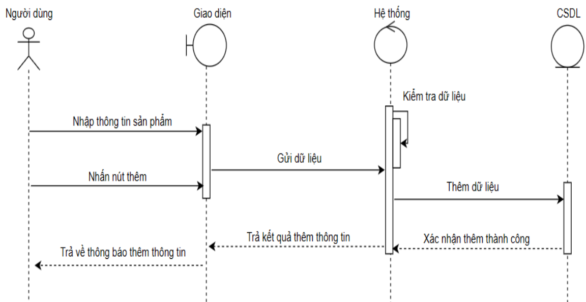
Hình 8: Sơ đồ trình tự thêm thông tin sản phẩm
