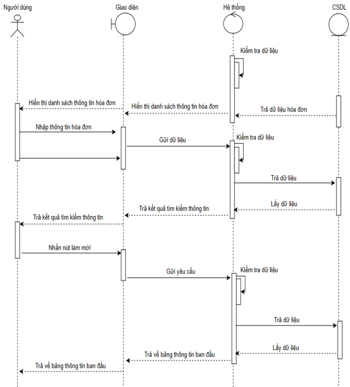
Hình 16: Sơ đồ trình tự xem hóa đơn
