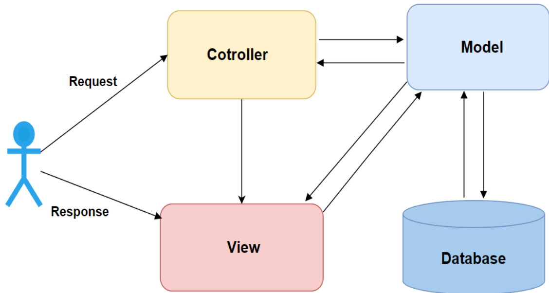
Hình 2: Sơ đồ kiến trúc MVC
