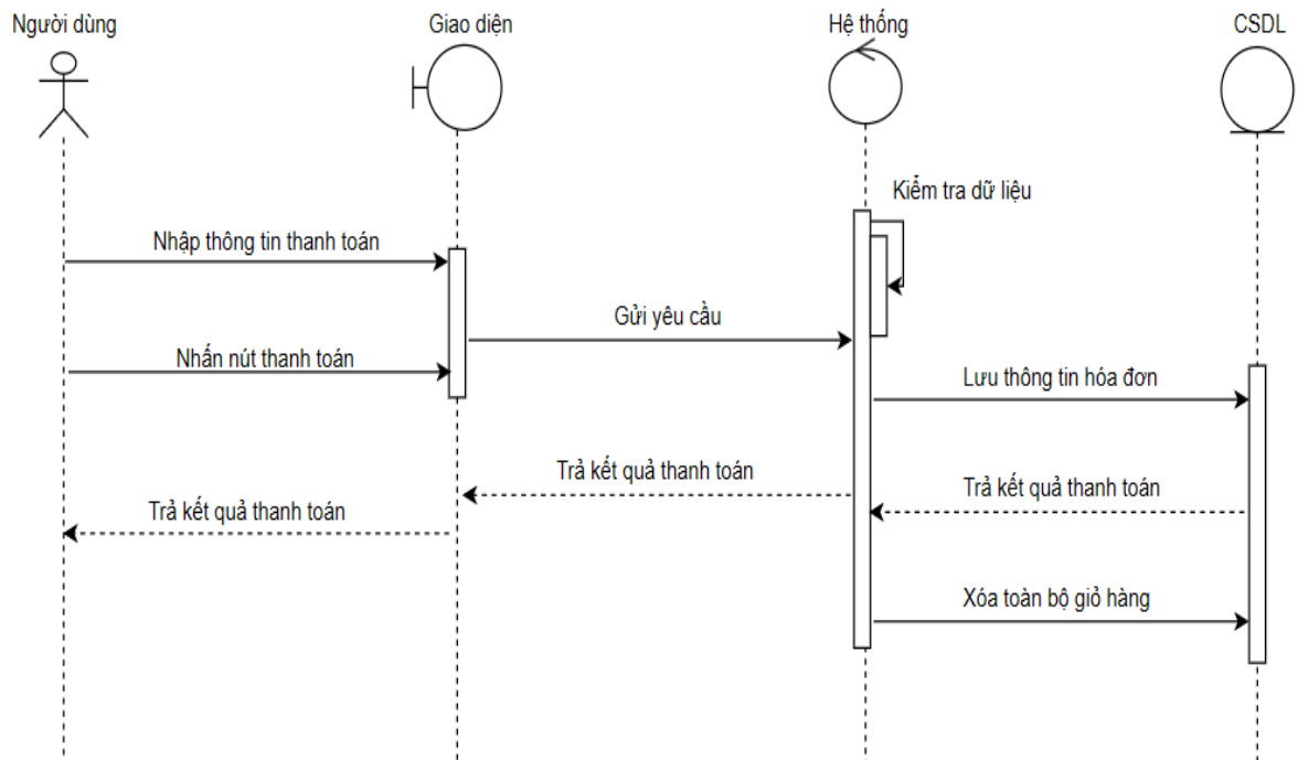
Hình 13: Sơ đồ trình tự thanh toán
