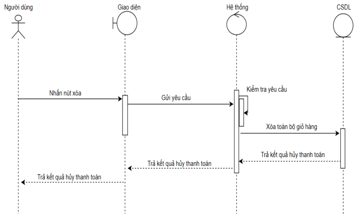
Hình 14: Sơ đồ trình tự hủy thanh toán
