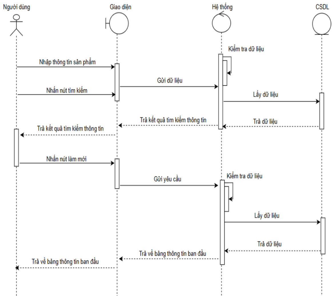
Hình 11: Sơ đồ trình tự tìm kiếm thông tin sản phẩm
