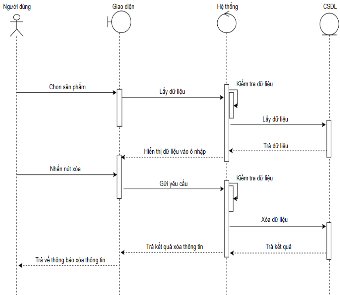
Hình 10: Sơ đồ trình tự xóa thông tin sản phẩm
