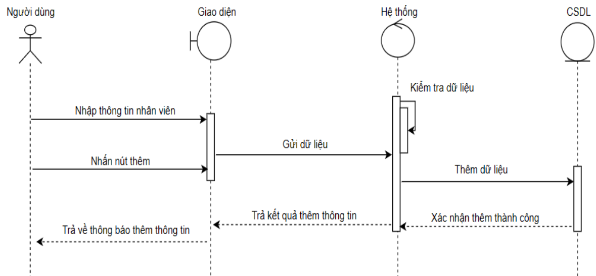
Hình 17: Sơ đồ trình tự thêm thông tin nhân viên
