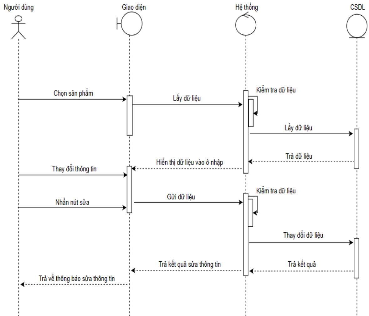
Hình 9: Sơ đồ trình tự sửa thông tin sản phẩm
