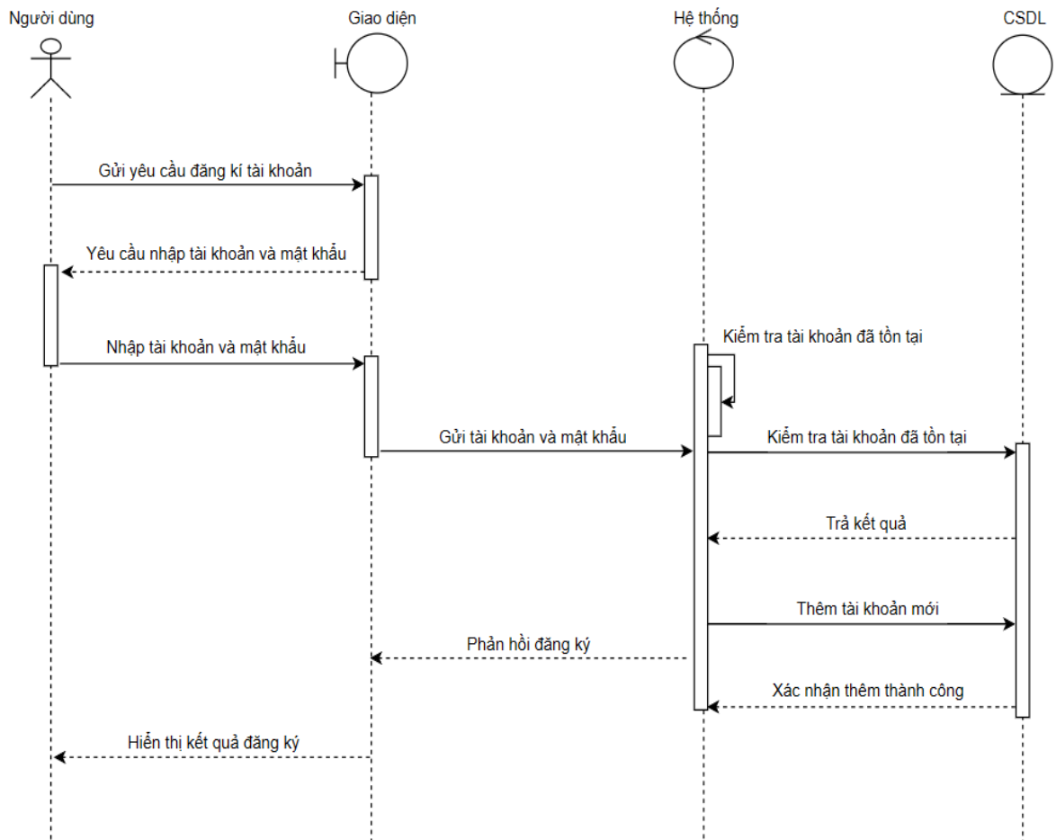
Hình 5: Sơ đồ trình tự đăng ký
