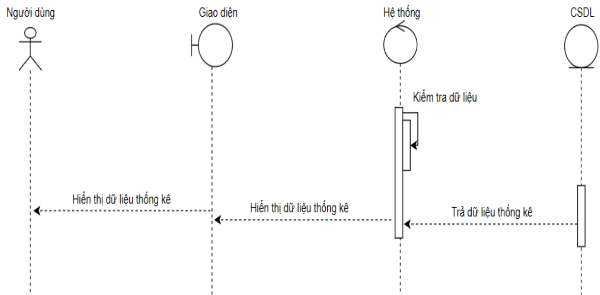
Hình 21: Sơ đồ trình tự thống kê
