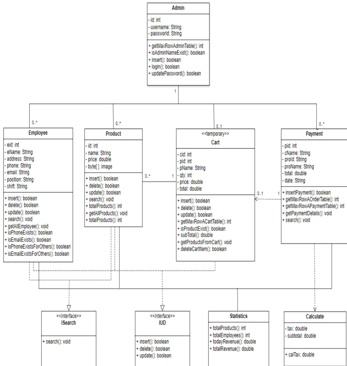
Hình 3: Sơ đồ lớp (Class Diagram)
