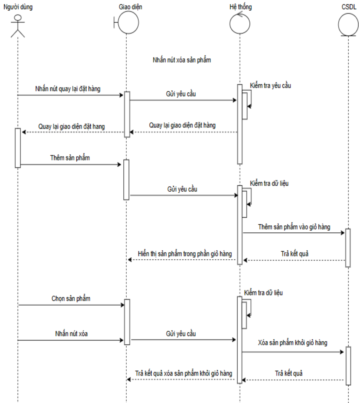
Hình 15: Sơ đồ trình tự thêm / bớt sản phẩm
