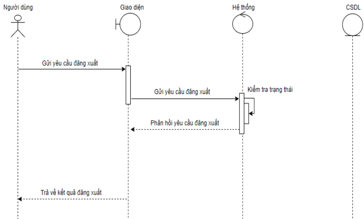
Hình 7: Sơ đồ trình tự đăng xuất
