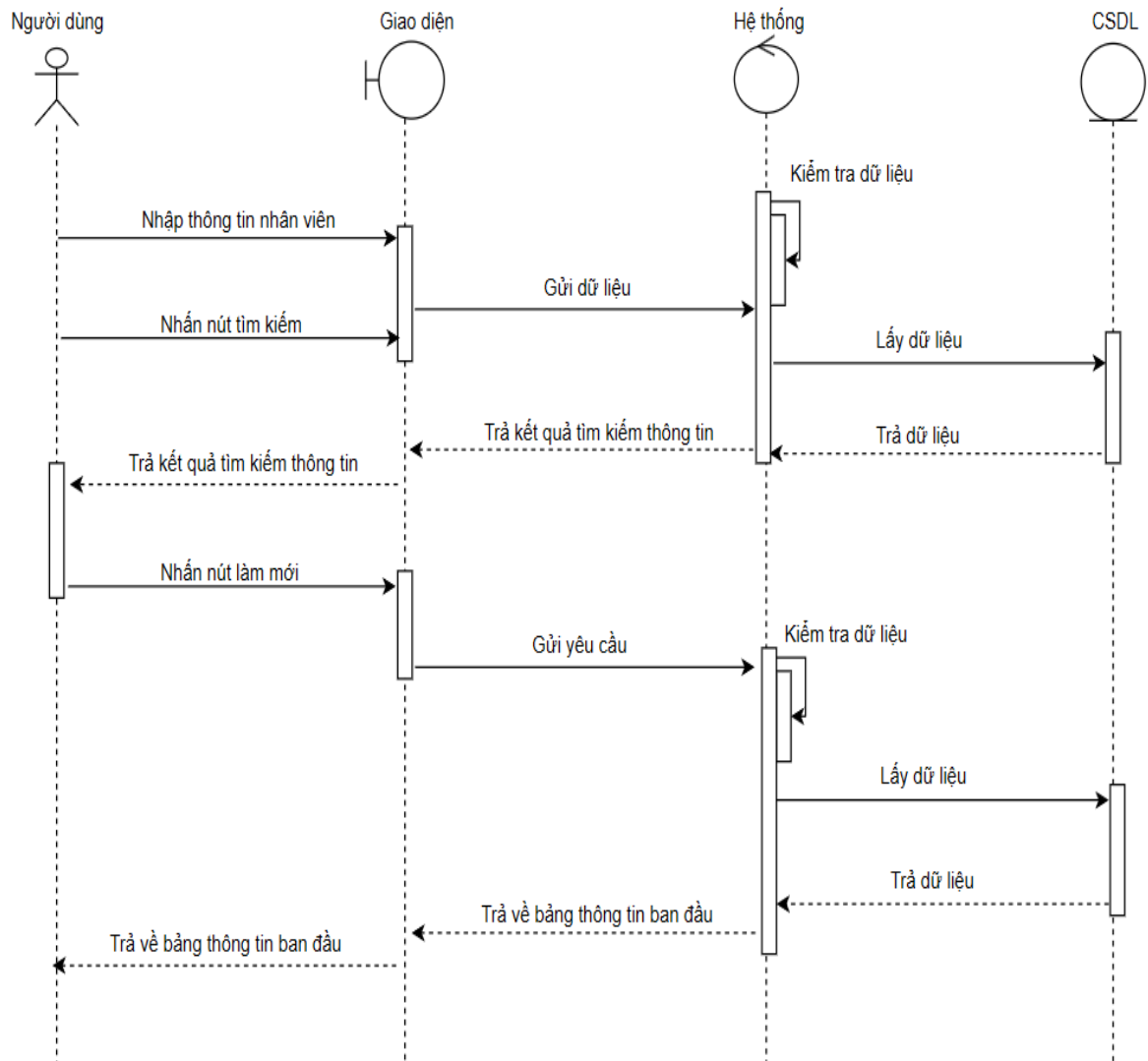
Hình 20: Sơ đồ trình tự tìm kiếm thông tin nhân viên
