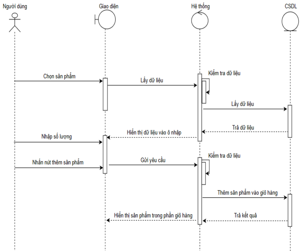
Hình 12: Sơ đồ trình tự thêm sản phẩm
